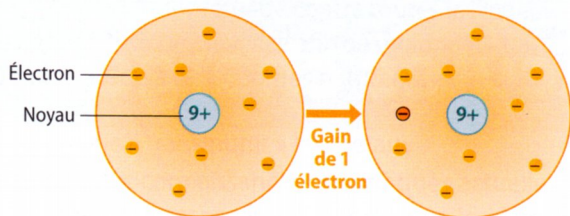
Fig. 1a : Atome de fluor.
