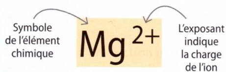
Fig. 3 : Formule de l'ion magnésium.
