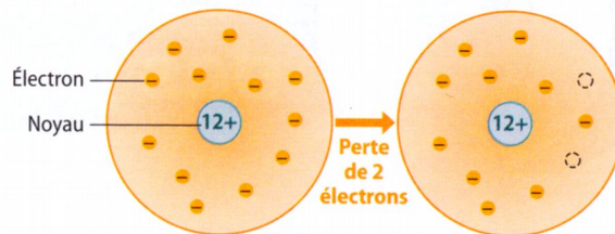
Fig. 2a : Atome de magnésium.
