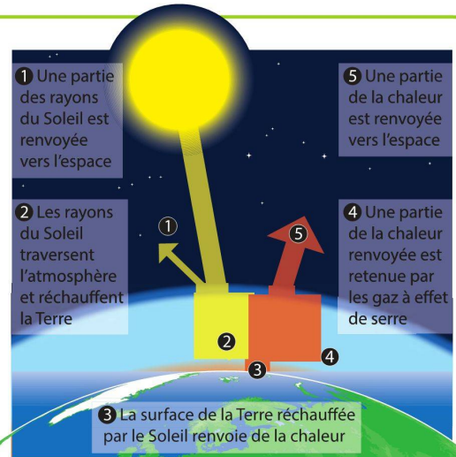
Fig. 1 : L'effet de serre naturel.
