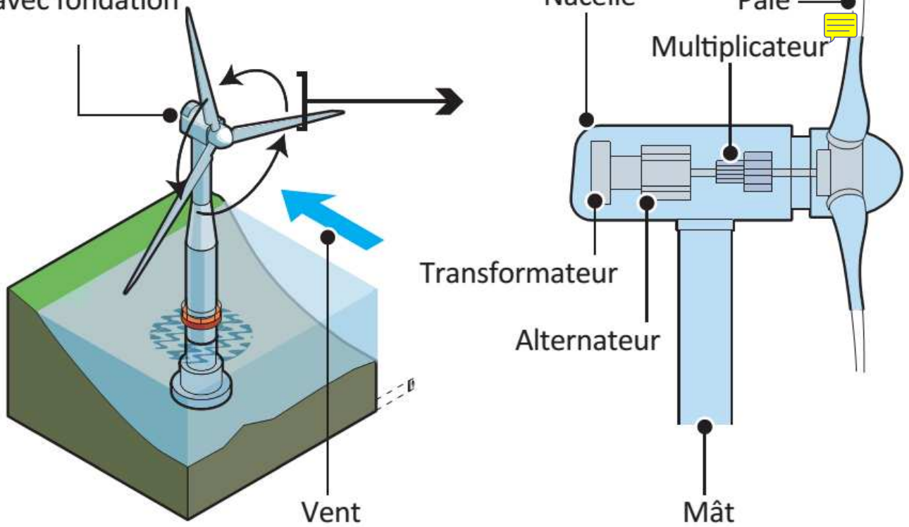
Eolienne classique avec fondation
